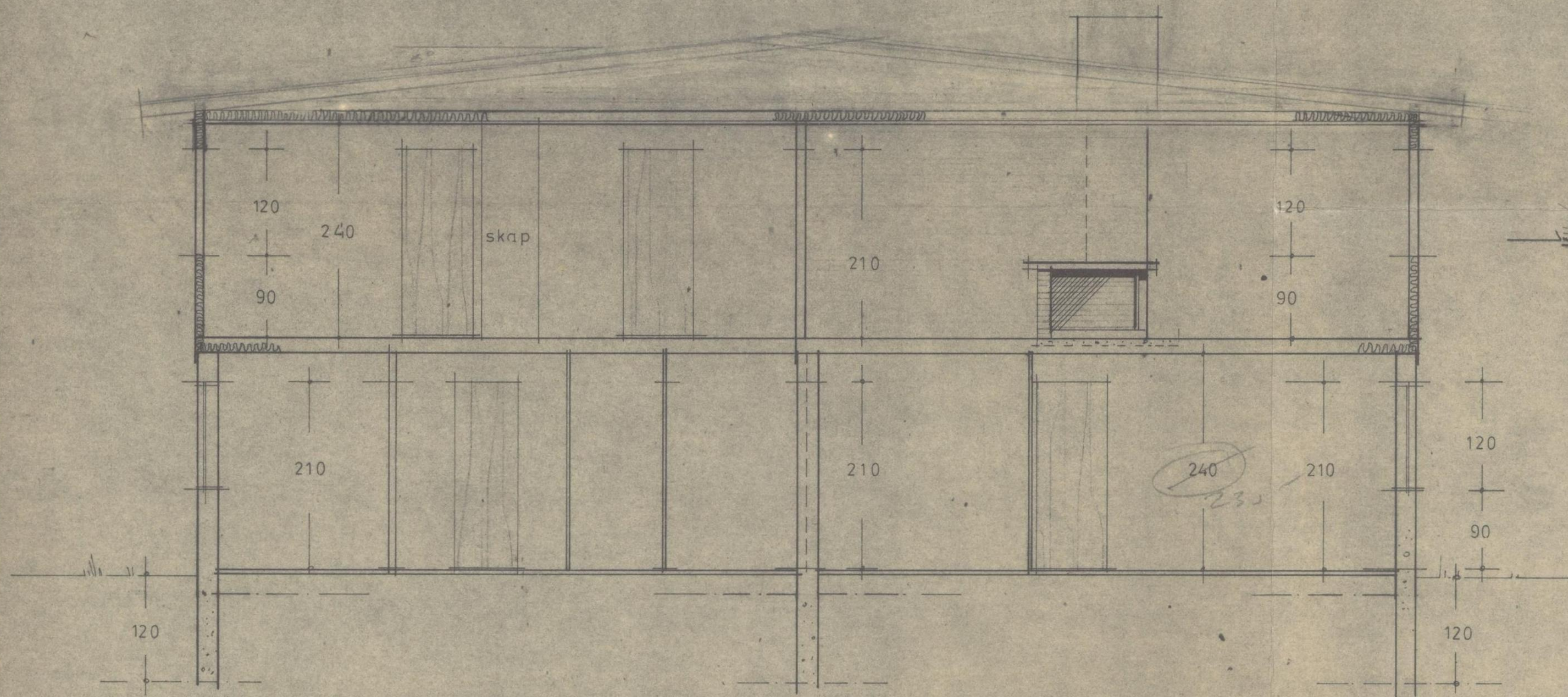
SNITT
